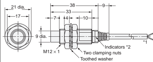
Diagram 6 E2E-X8MD□ E2E-X5ME□/F□
