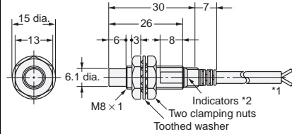
Diagram 2 E2E-X4MD□ E2E-X2ME□/F□
