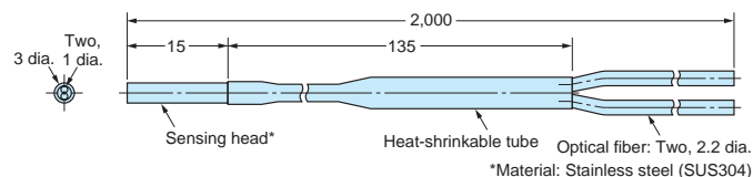
E32-D12 E32-D12R
