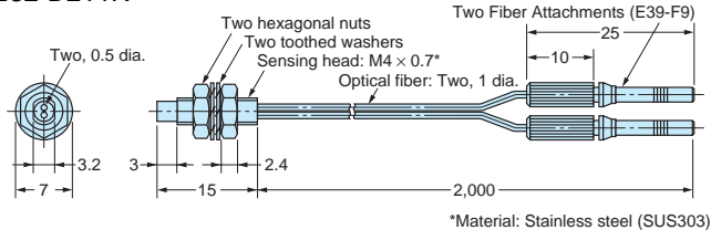
E32-DC200E E32-D21R
