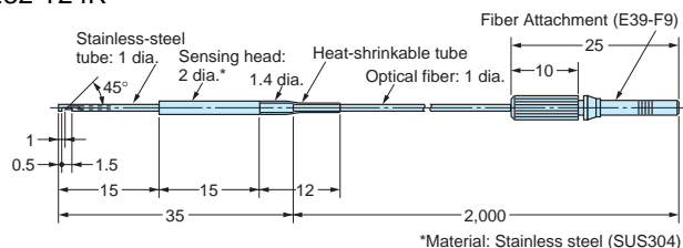
E32-T24 E32-T24R
