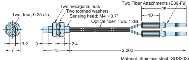
E32-D221B
