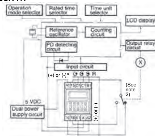
H3CA-FA
