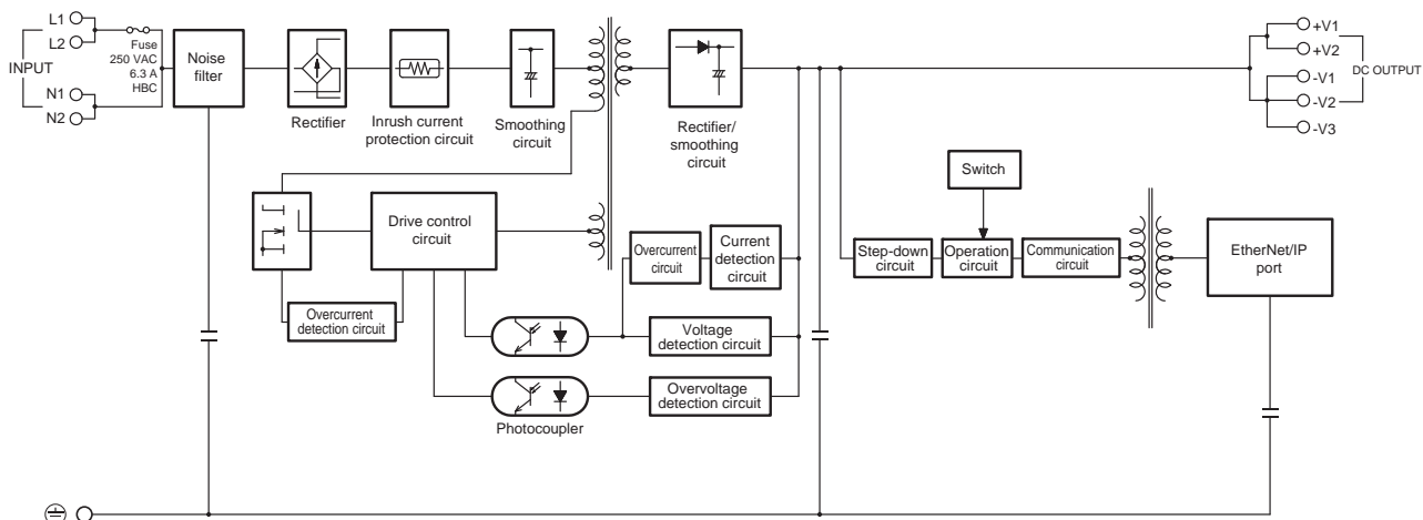
S8VK-X09024-EIP
